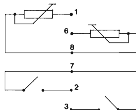
Rys. 2. Schemat elektryczny zespołu wioselek.
