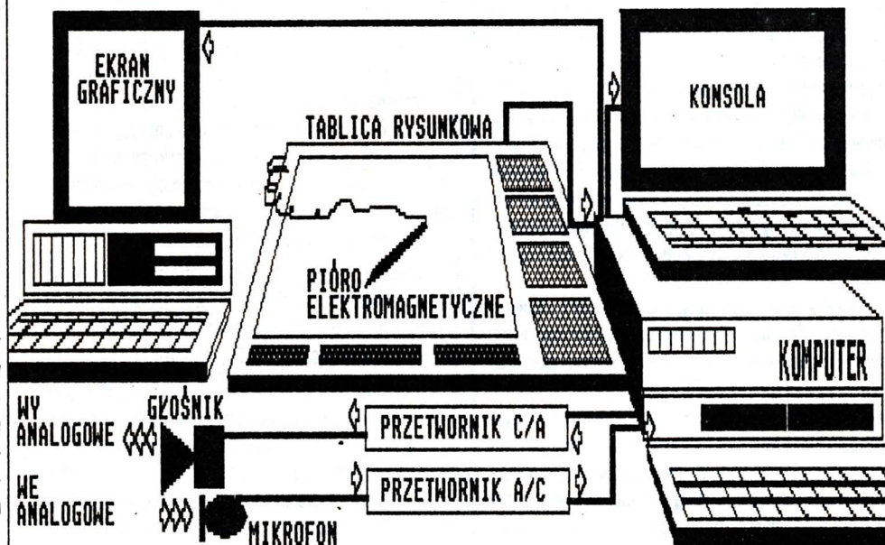
Rys. 1 Podstawowa konfiguracja systemu UPIC
