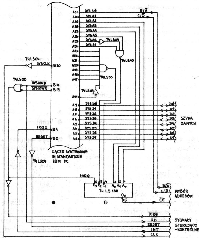
Rys. 2 Metoda przyłączenia interfejsu MIDI do komputera w standardzie IBM PC
