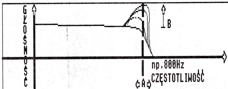
Rys. 2A Wykres graficzny przedstawiający pracę filtra dolnoprzepustowego
