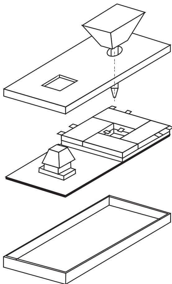
Rys. 4. Drążek sterowy, sposób montażu
