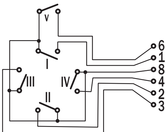
Rys. 6. Schemat elektryczny, układ drążka
