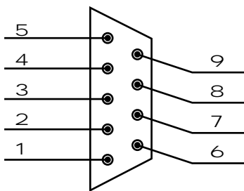
Rys. 1. Połączenie PORT A z gniazdami joysticków.
