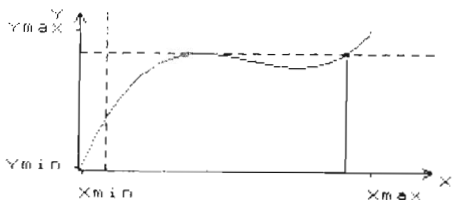
PRZEBIEG FUNKCJI y = x^3 + x^2 - 9x + 24 - 20
