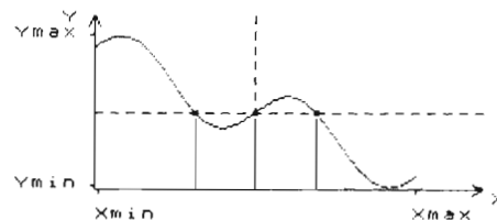
PRZEBIEG FUNKCJI y = \sin x - x/3
